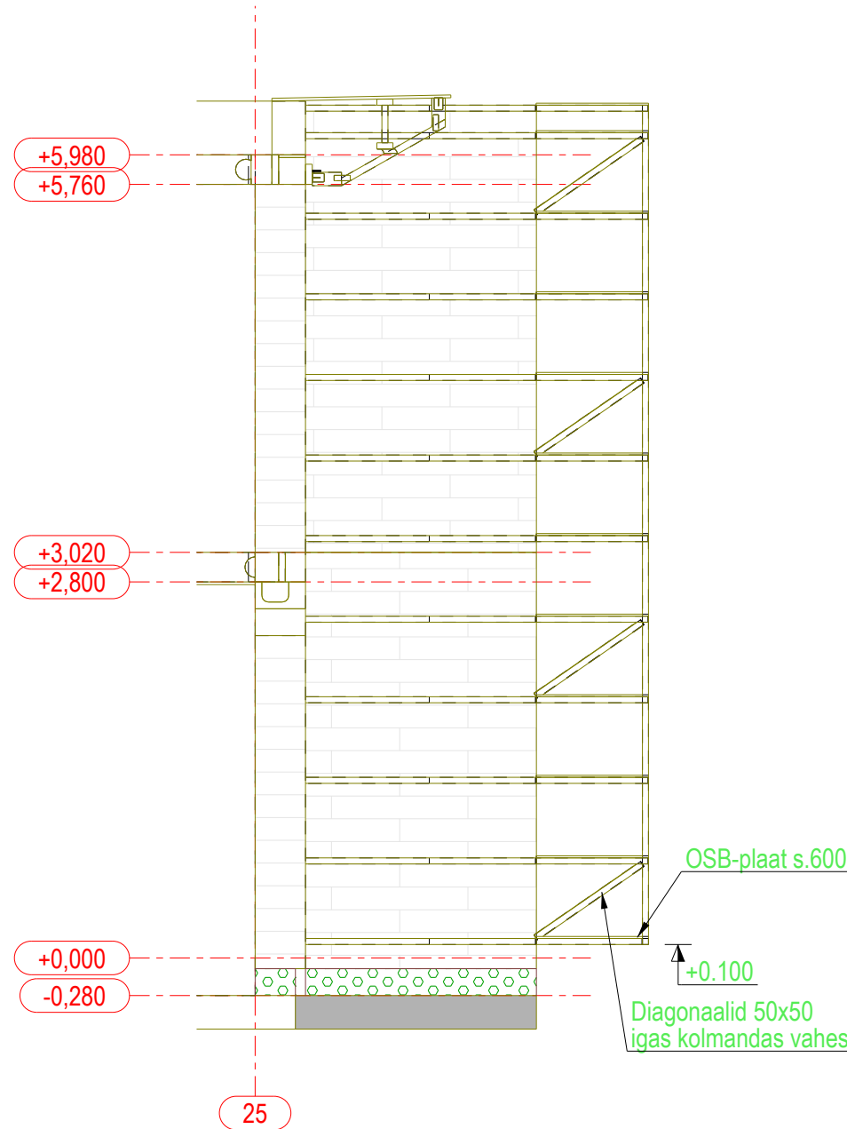
A-A 1:50
