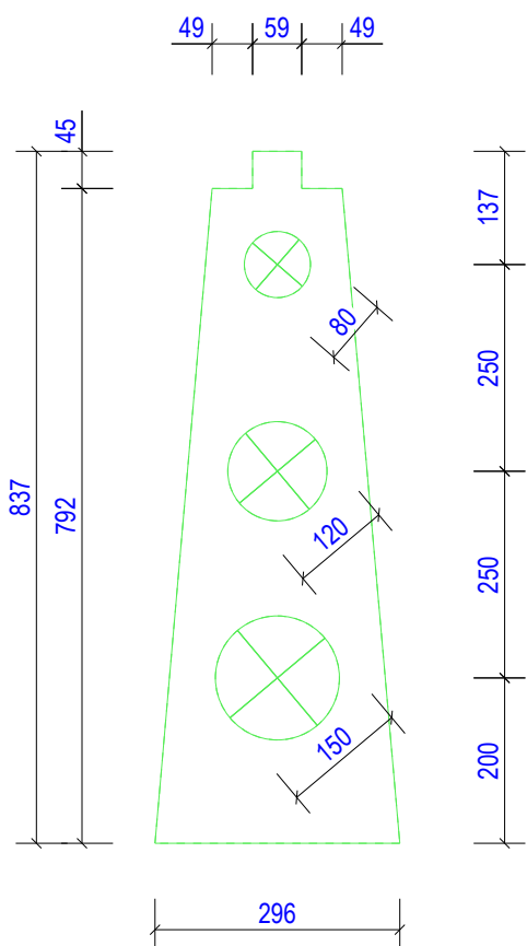
OSB-plaadi kuju 1:10
